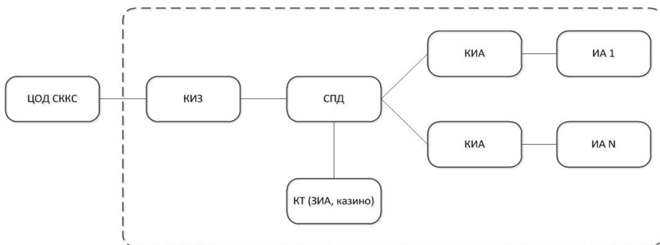
Рисунок 2. Структурная схема подсистемы подключения ЗИА и казино
