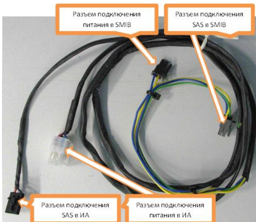
Рисунок 3.4.2 – Кабель соединительный IGT 05-10
