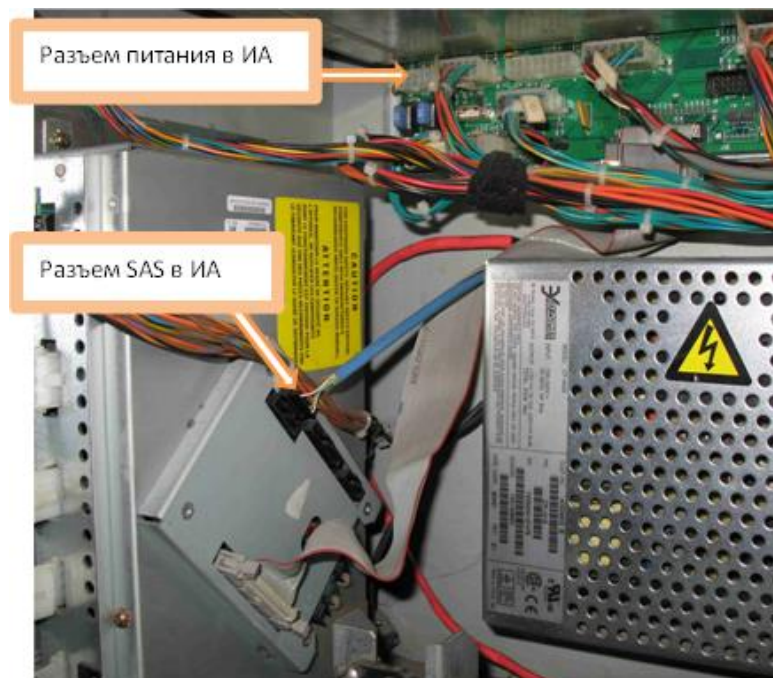
Рисунок 3.4.1 – Месторасположение переходных плат ИА.
