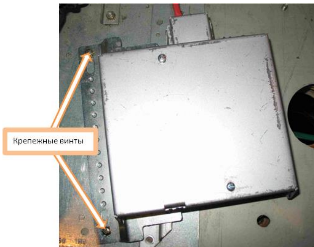
Рисунок 3.3.1 – Закреплённый КИА в ИА
