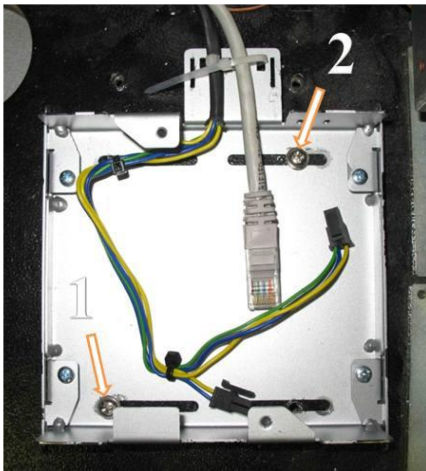
Рисунок 3.3.1 Крепление КИА
