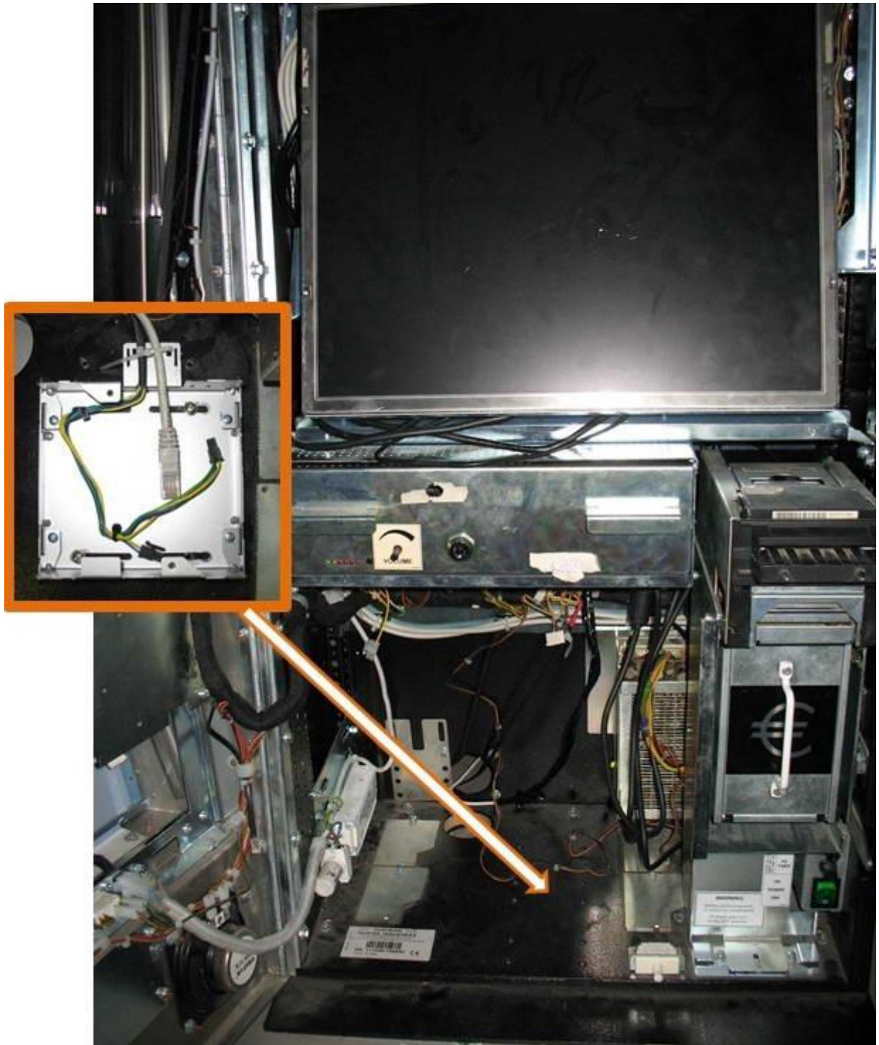
Рисунок 3.1.1 Месторасположение КИА (фронтальный вид ИА)
