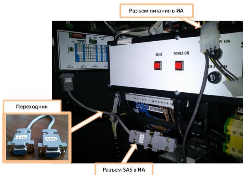
Рисунок 3.4.1 – Подключение соединительного кабеля в ИА.
