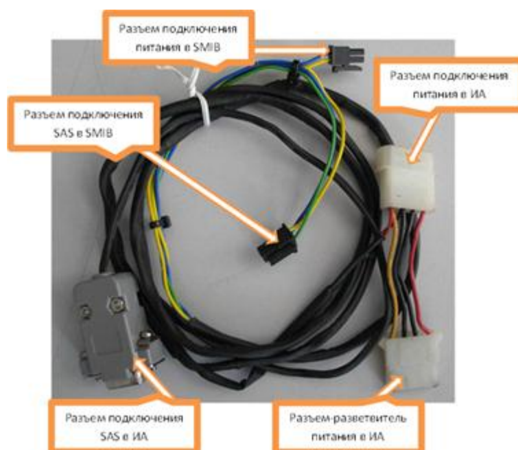
Рисунок 3.4.2 – Кабель соединительный RuI 09M-04
