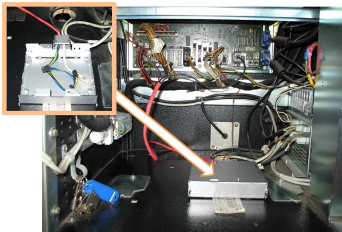
Рисунок 3.1.1 Месторасположение КИА (фронтальный вид ИА)
