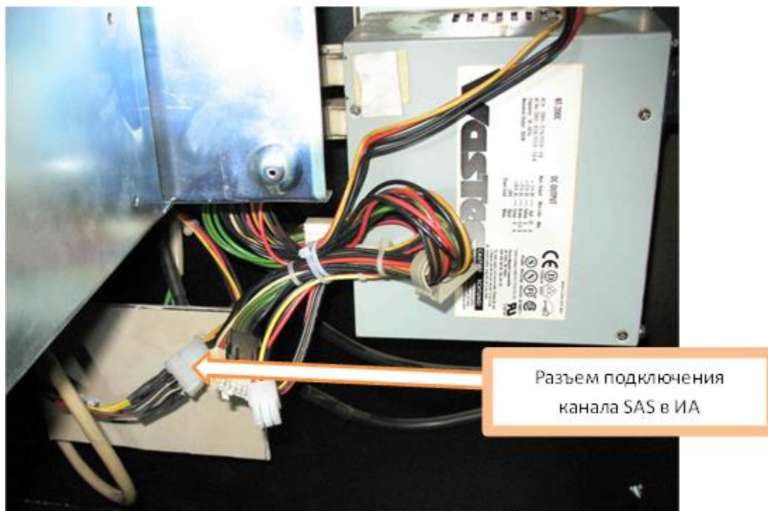
Рисунок 3.4.2 – Подключение питания в ИА
