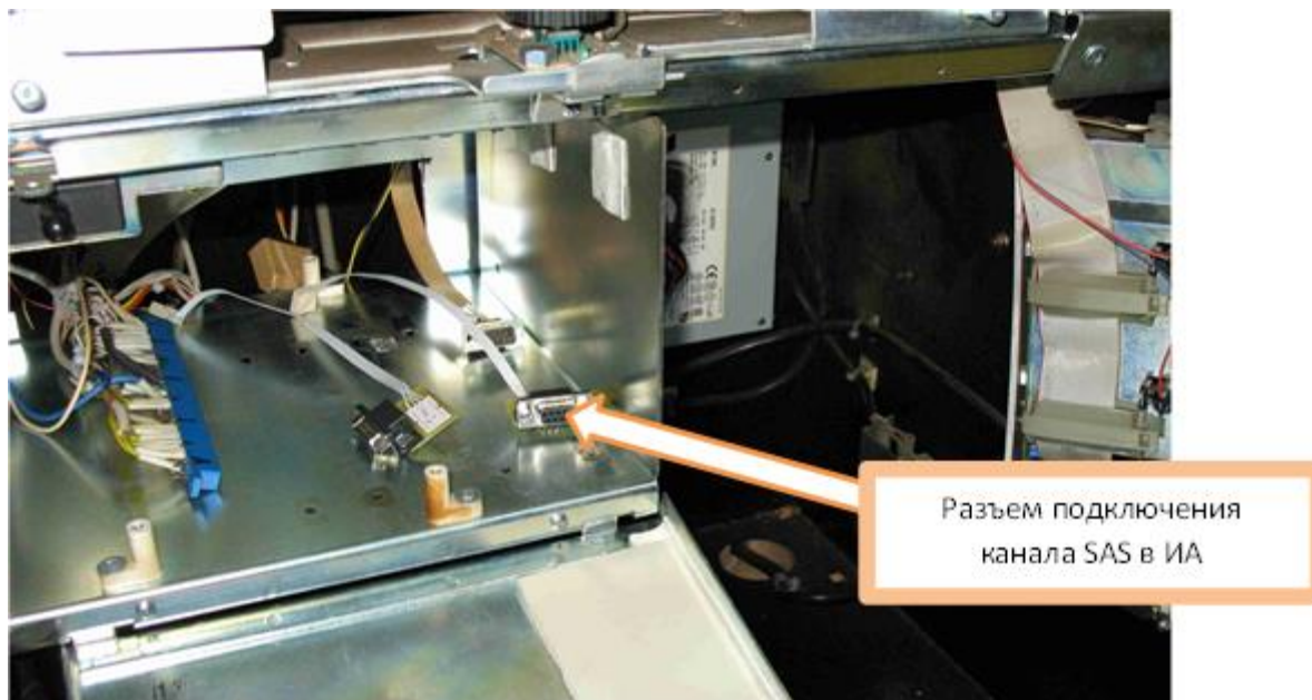
Рисунок 3.4.1 – Подключение канала SAS в ИА.
