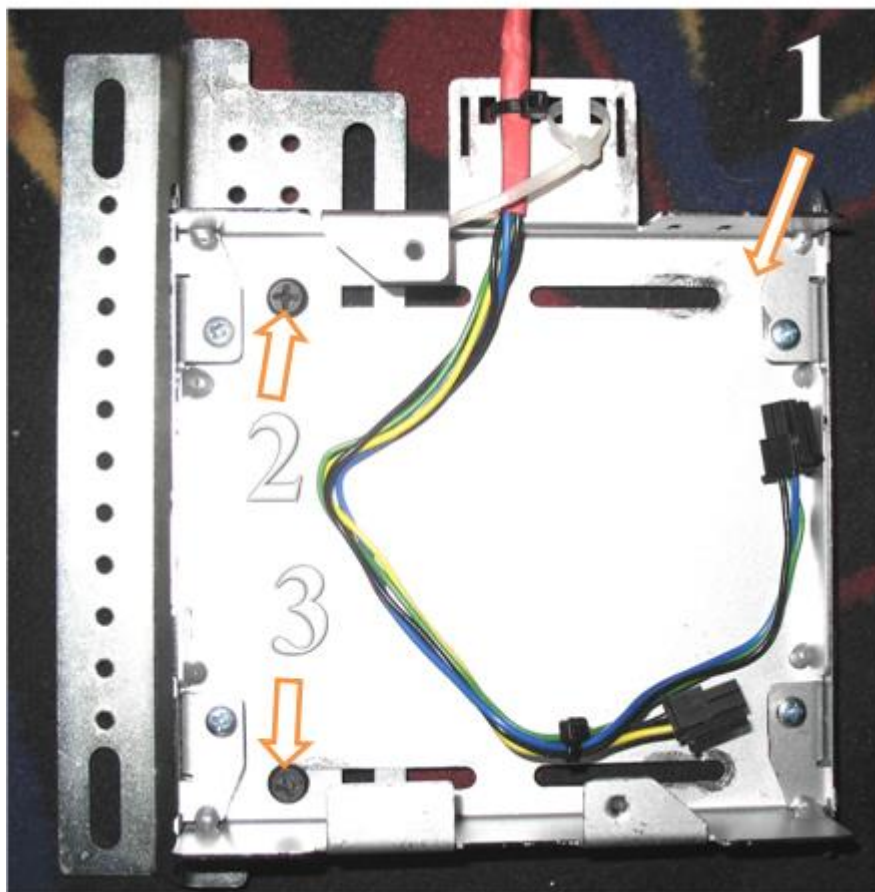
Рисунок 3.2.1 Установка кронштейна платформы КИА
