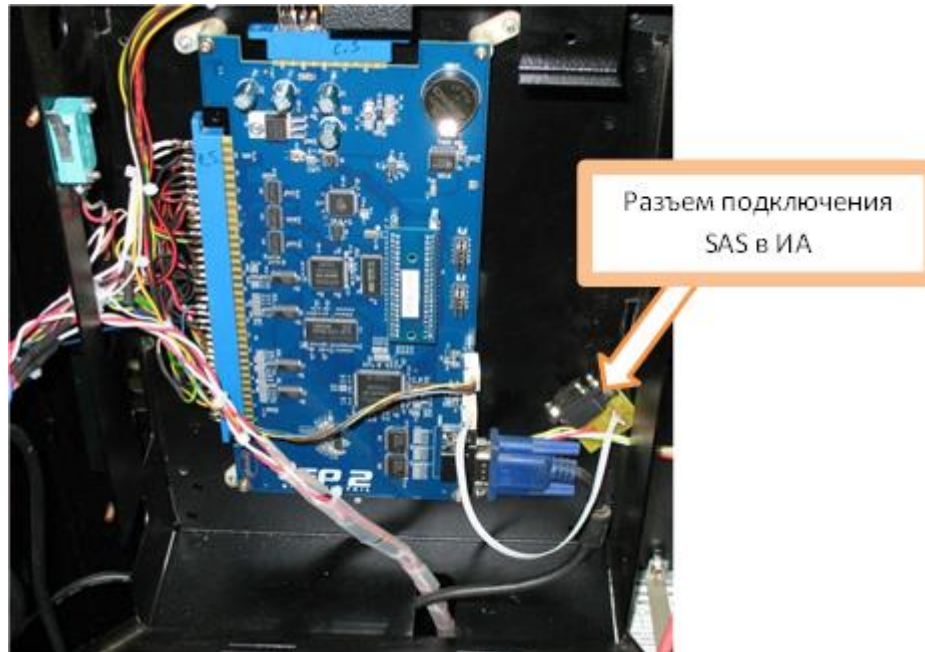
Рисунок 3.4.1 – Подключение канала SAS в ИА.
