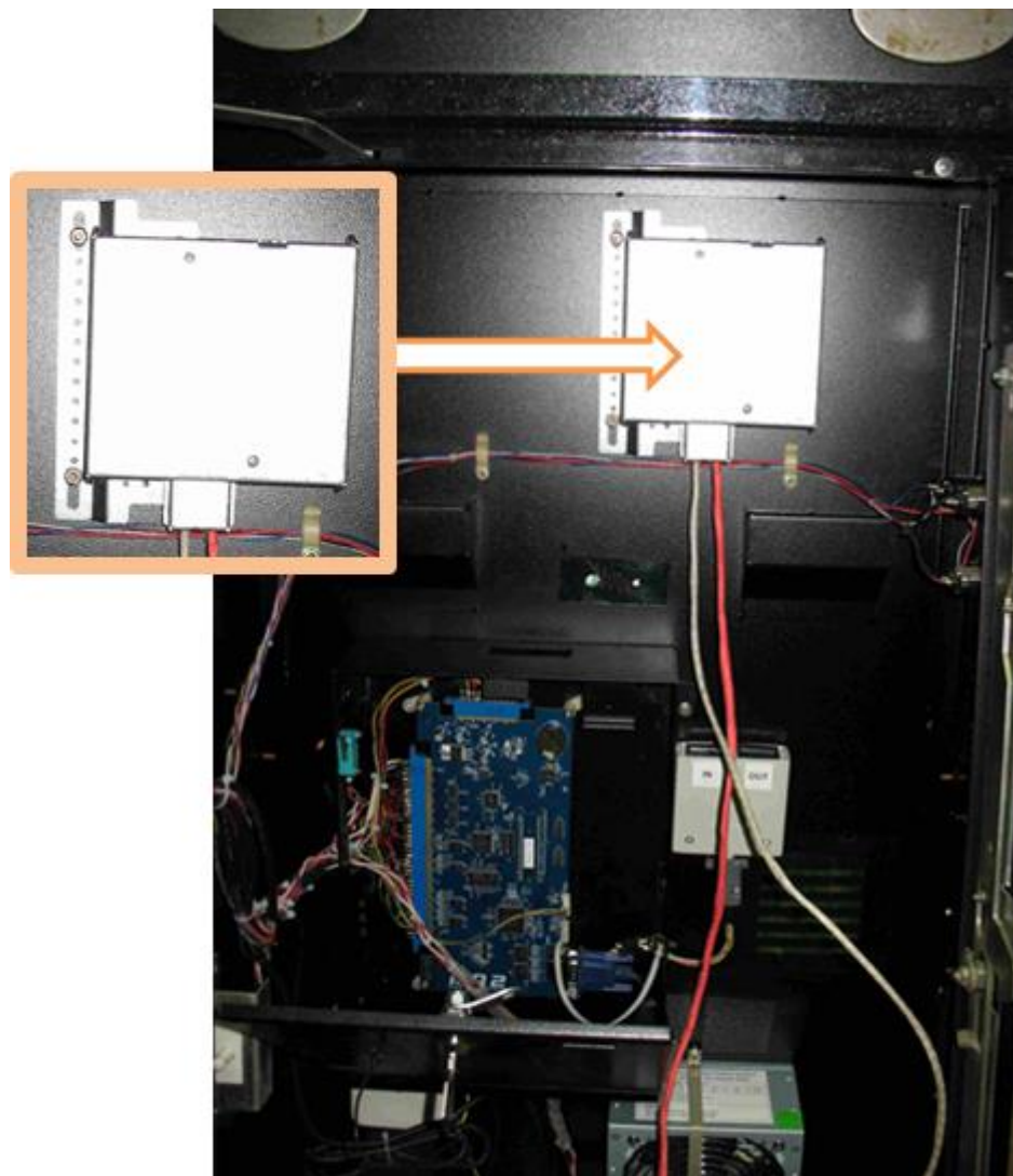
Рисунок 3.1.1 Месторасположение КИА (фронтальный вид ИА)
