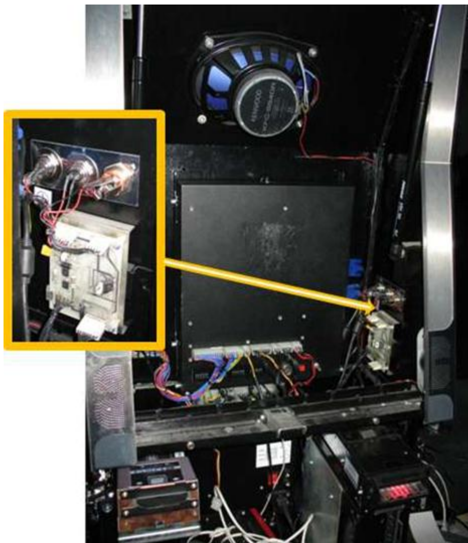
Рисунок 3.1.1. Месторасположение КИА (фронтальный вид ИА)
