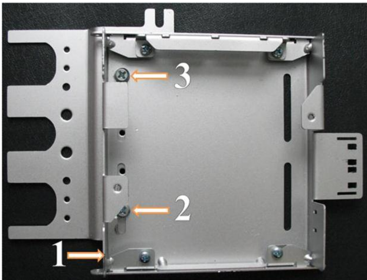
Рисунок 3.2.1 Установка кронштейна крепления платформы КИА
