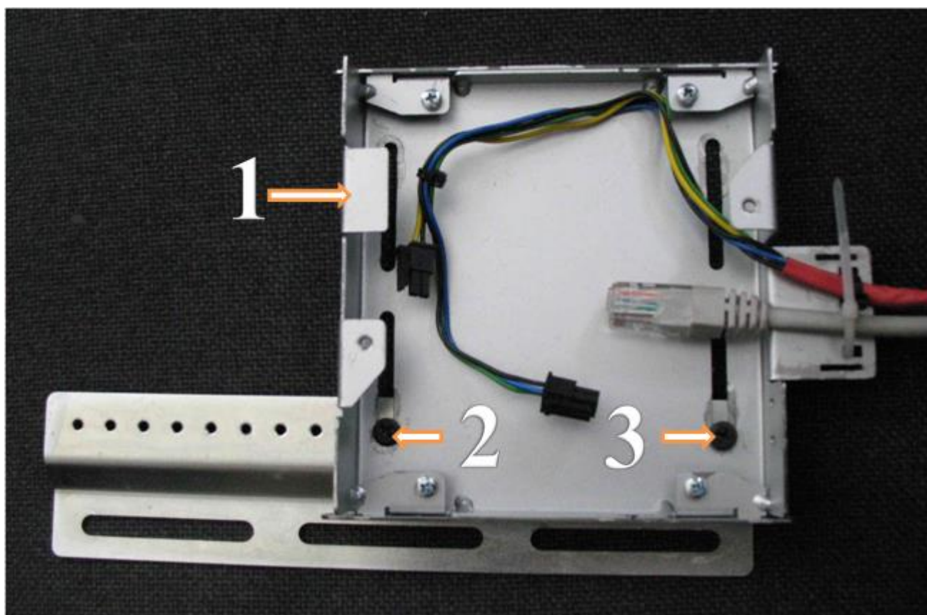
Рисунок 3.2.1 Установка кронштейна платформы КИА
