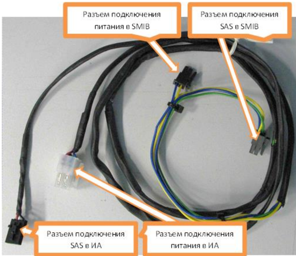
Рисунок 3.4.3 – Кабель соединительный IGT 05-10
