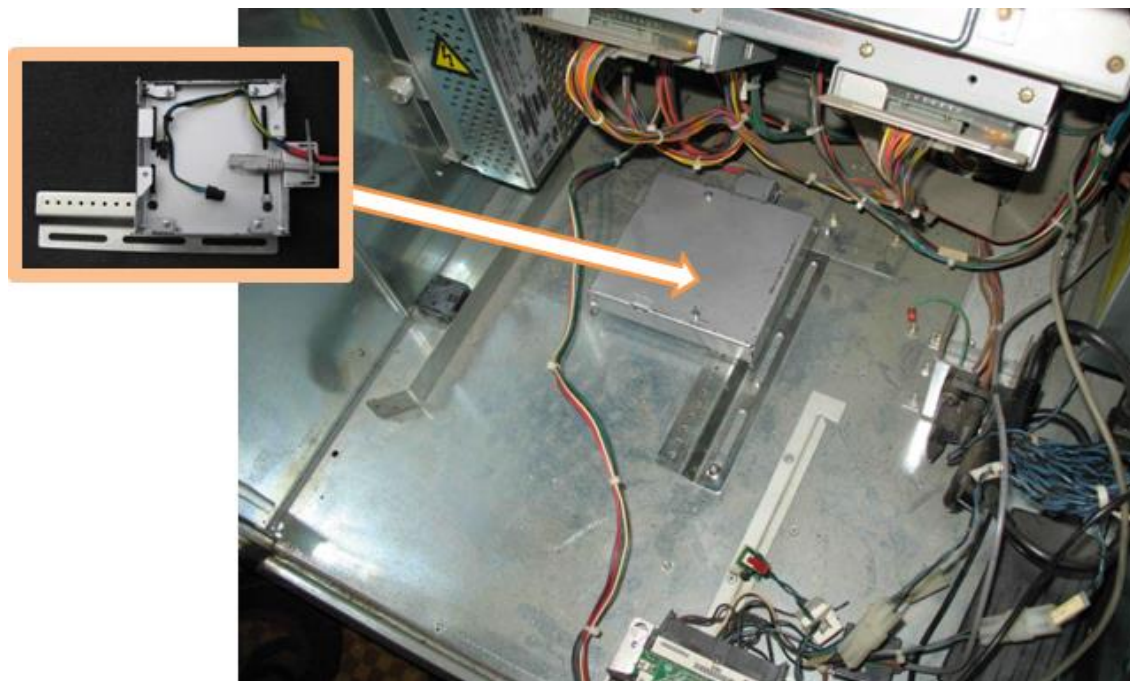
Рисунок 3.1.1 Месторасположение КИА (фронтальный вид ИА)
