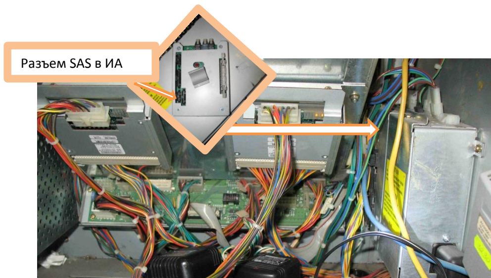
Рисунок 3.4.2 – Подключение канала SAS в ИА.
