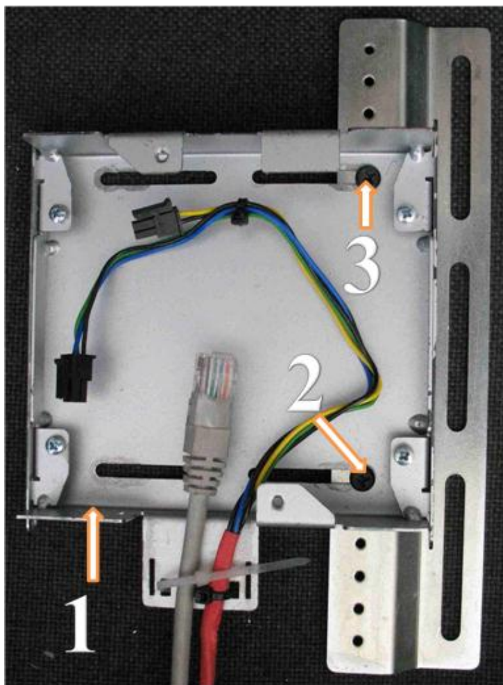
Рисунок 3.2.1 Установка кронштейна платформы КИА
