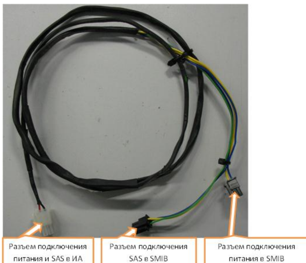
Рисунок 3.4.2 – Кабель соединительный Veg 04
