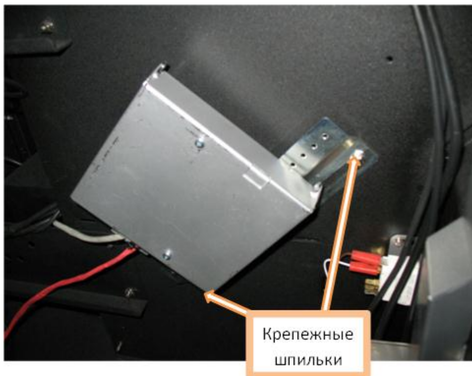
Рисунок 3.3.1 – Закреплённый КИА в ИА
