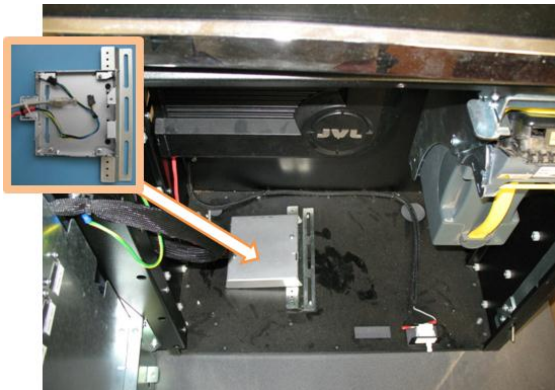
Рисунок 3.1.1 Месторасположение КИА (фронтальный вид ИА)
