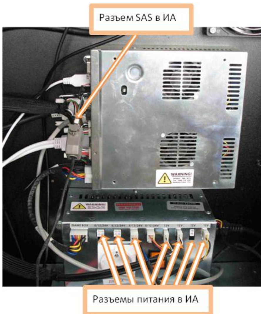
Рисунок 3.4.1 –Подключение питания КИА и канала SAS.
