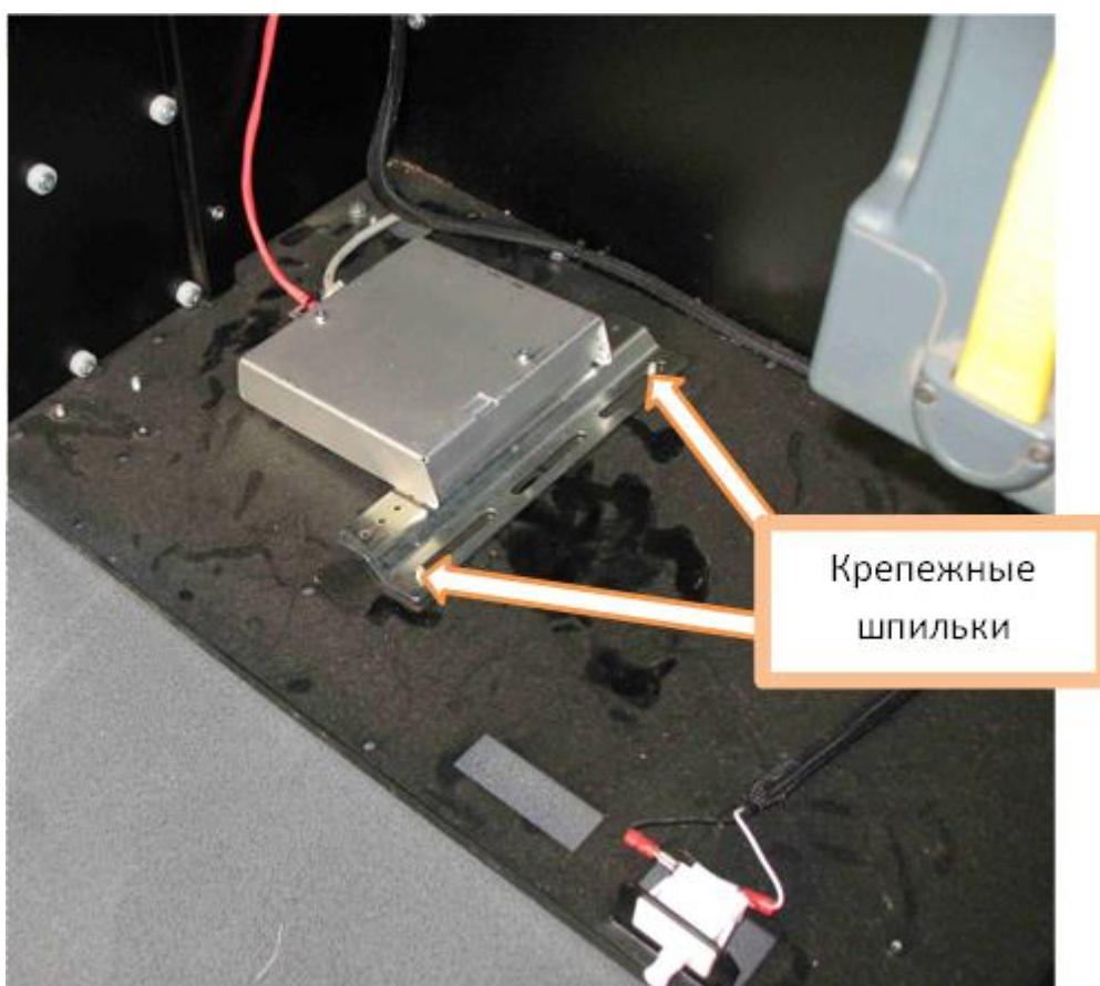
Рисунок 3.3.1 – Закреплённый КИА в ИА
