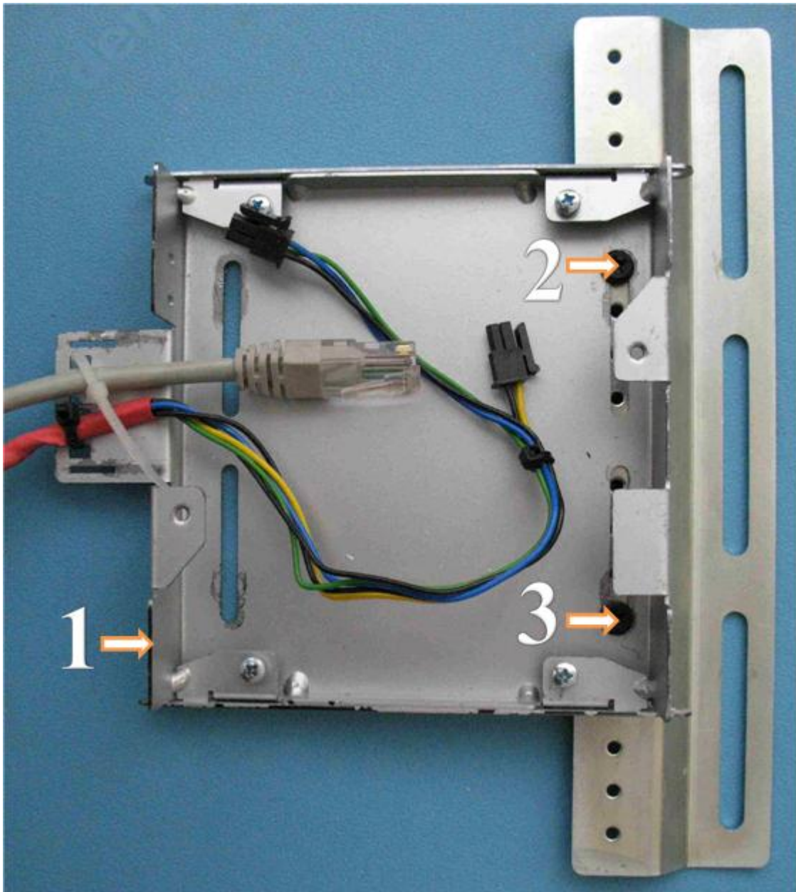
Рисунок 3.2.1 Установка кронштейна платформы КИА
