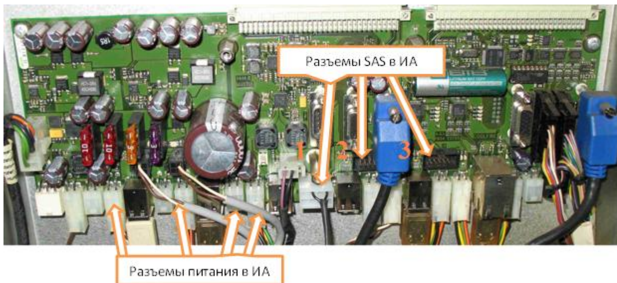
Рисунок 3.4.1 – переходная плата ИА.
