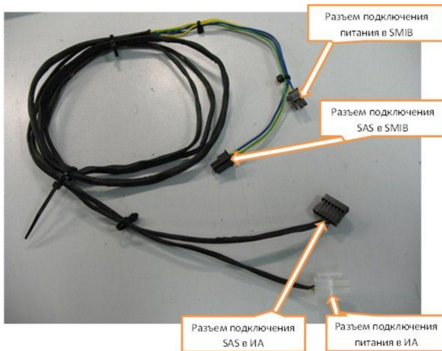
Рисунок 3.4.3 – Кабель соединительный Nov 10-04
