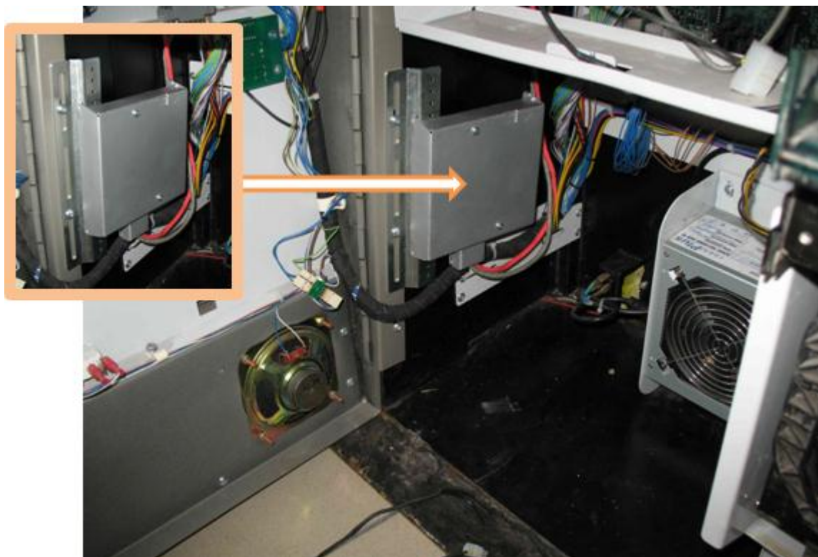
Рисунок 3.1.1 Месторасположение КИА (фронтальный вид ИА)
