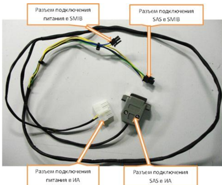
Рисунок 3.4.2 – Кабель соединительный Nov 15-12
