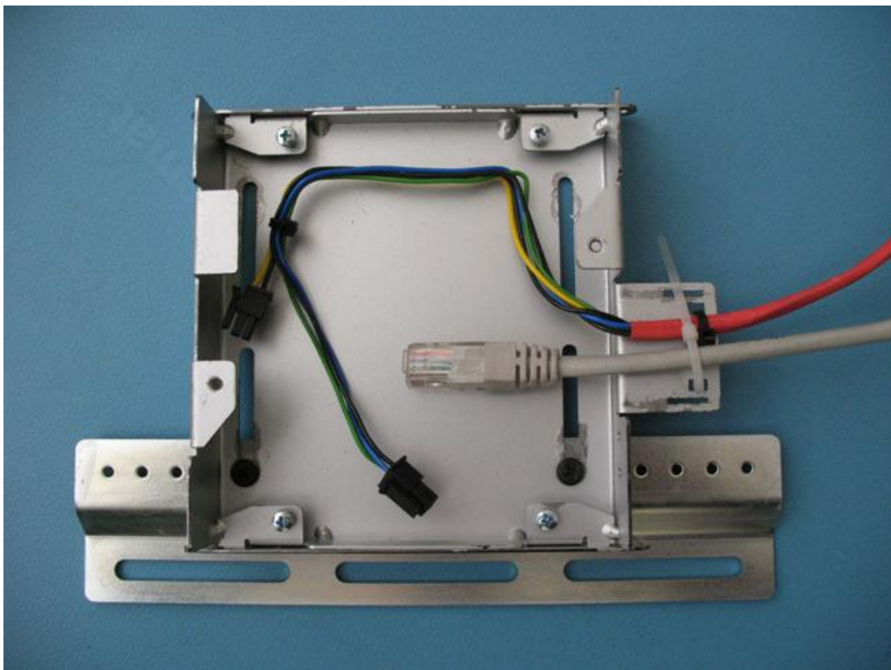
Рисунок 3.2.1 Установка кронштейна платформы КИА
